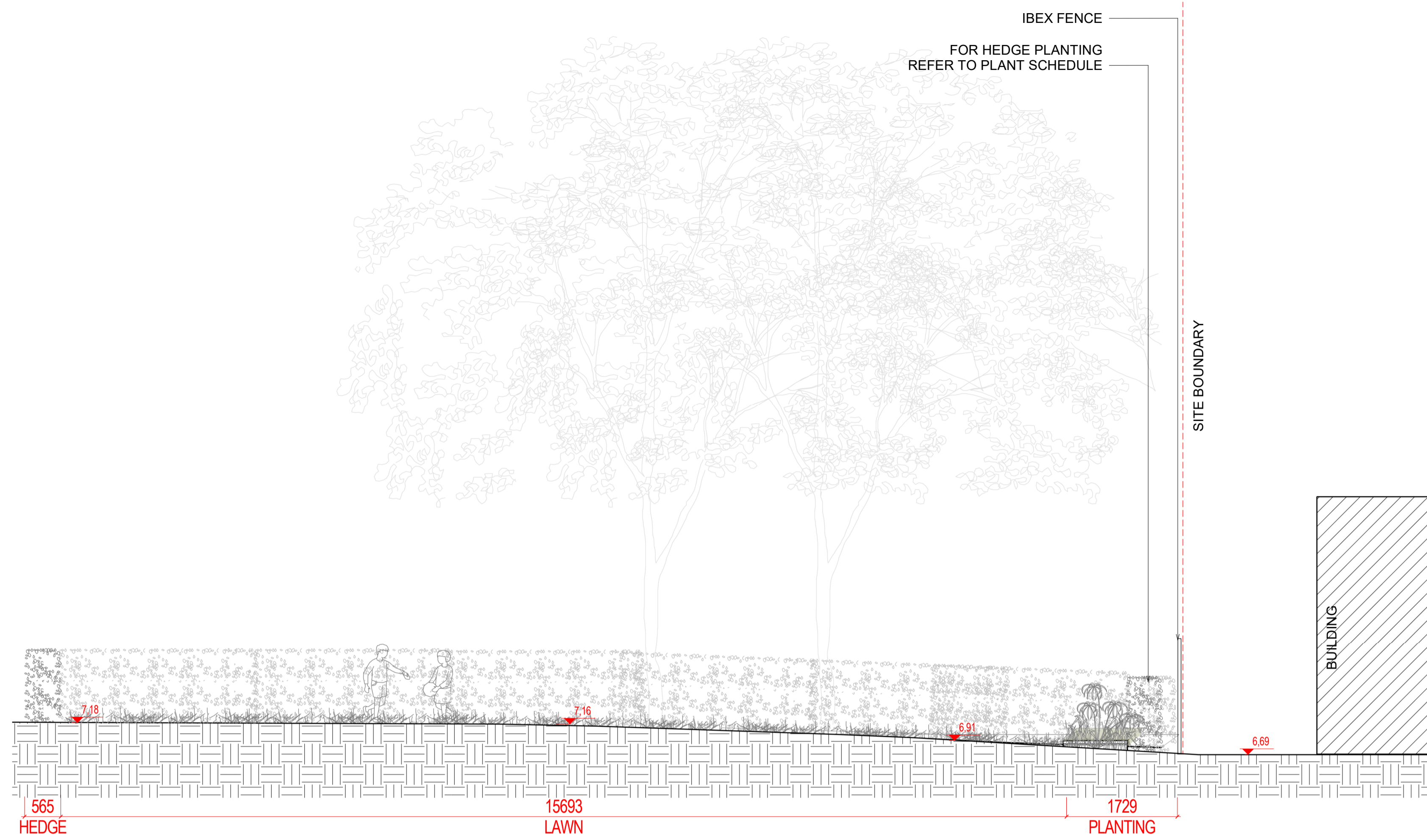
1 SECTION 05 1:50 @A1
